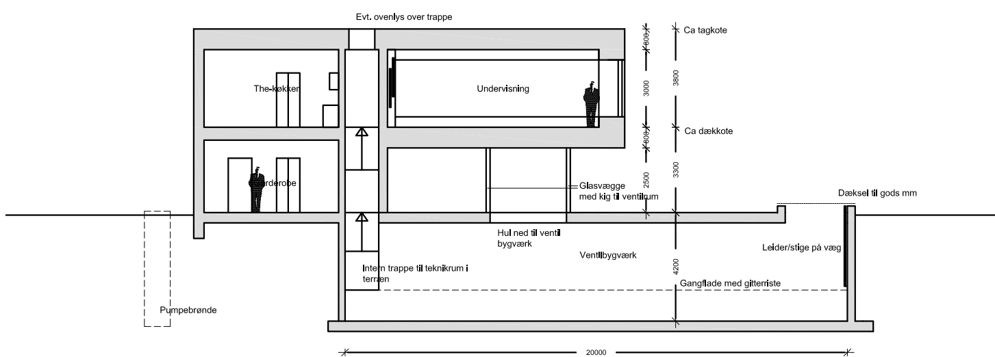
Længdesnit
