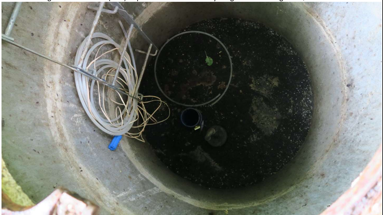
Foto 44: Boring DGU. Nr. 81.135 (O21) ) er udført i Ø125 filterrør, placeret i Ø1500 betonringe med støbt bund og betonlåg med Ø60 mandehul.
