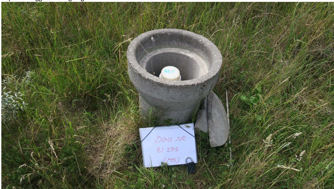
Foto 12: Boring DGU. Nr. 81.295 (M5) er udført i Ø125 filterrør, placeret i et Ø300 mufferrør, med betonlåg og låsestang.
