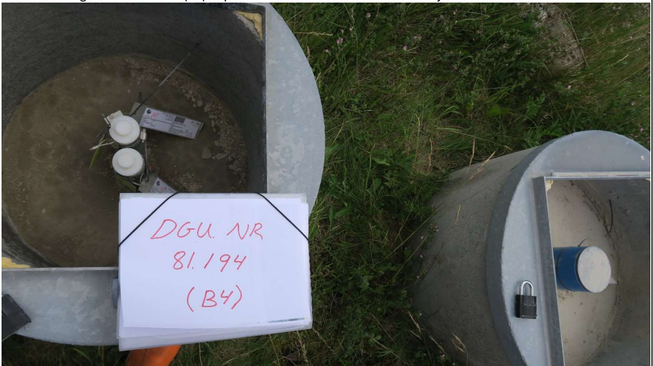
Foto 24: Boring DGU. Nr. 81.194 (B4) har 3 indtag, placeret i 2 stk. Ø600 betonrør med støbt bund og 50 cm firkantet galvaniseret låg. Indtag 1 er Ø125, Indtag 2 og indtag 3 er Ø63.
