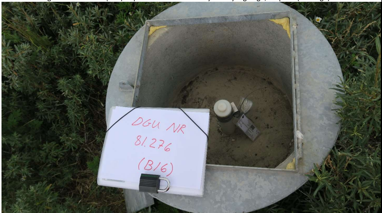
Foto 42: Boring DGU Nr. 81.276 (B16) ) er udført i Ø63 filterrør, placeret i Ø600 betonrør med støbt bund og 50 cm firkantet galvaniseret låg.
